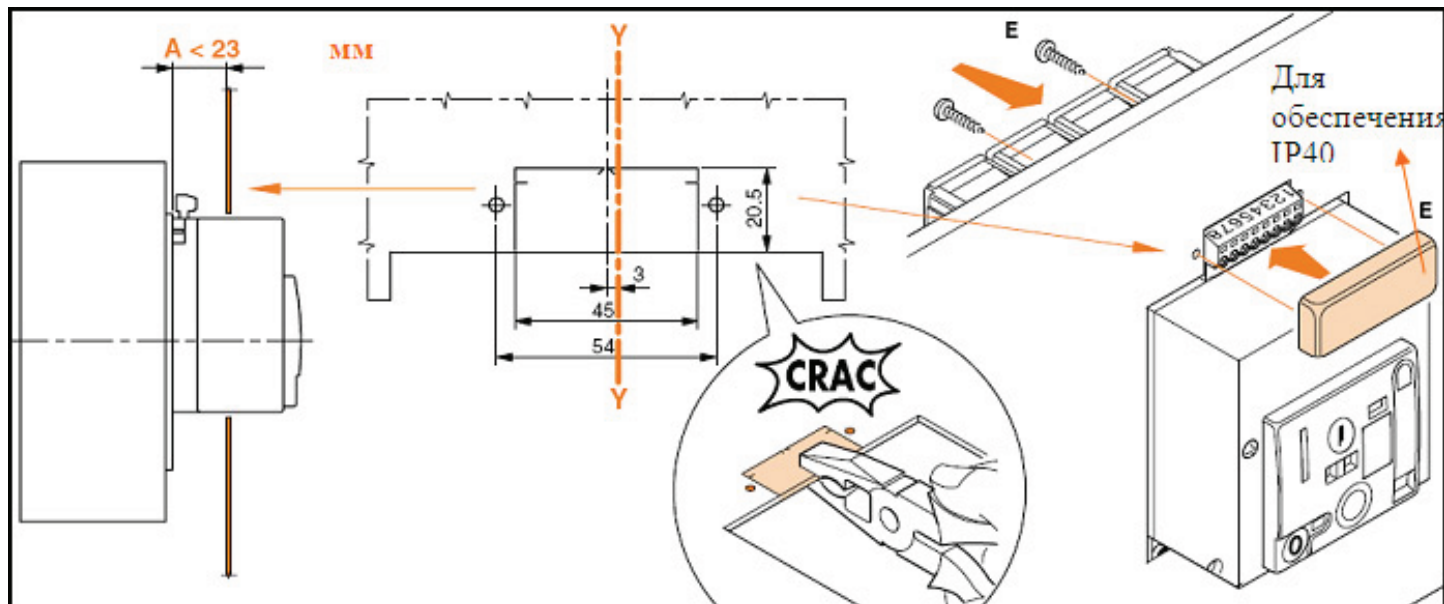
Рис. 3. Электродвигательный привод, смонтированный в панели щита
