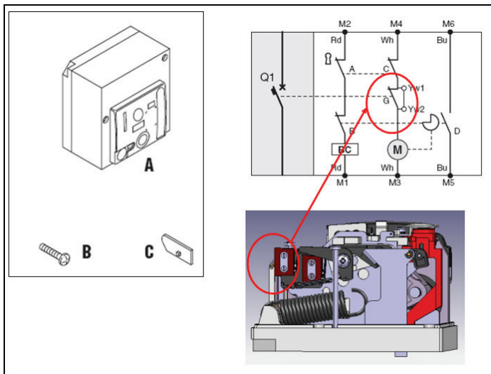
Рис. 1. Электродвигательный привод БЕЗ клеммного блока (выпущен до 41-й недели 2008 г.). Внешний вид, устройство и электрическая схема.
