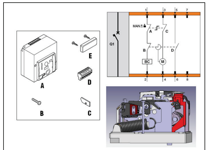
Рис. 2 - Новый электродвигательный привод DPX630 с клеммным блоком (выпускается с 41-й недели 2008 г.). Внешний вид, устройство и электрическая схема.
