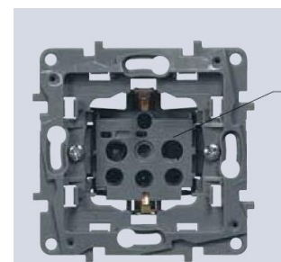
Обновленный механизм розетки 2К+3 ЕТИКА с защитными шторками
