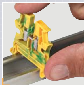
Безвинтовое крепление защитных клемм на DIN-рейке
