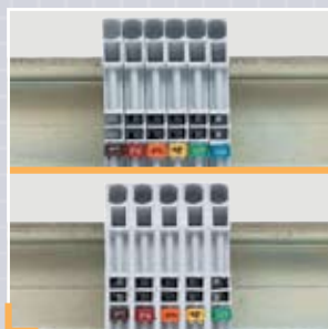
Выбор ширины 5 или 6 мм для сечения 4 мм 2 (I e = 32 A)
